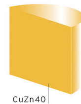
CuZn40
